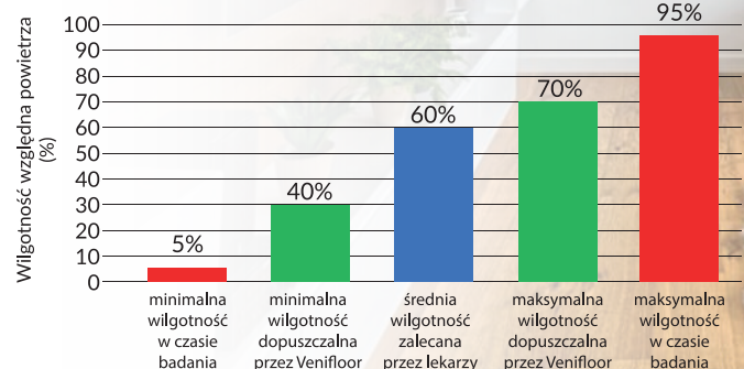
Rys. Wilgotność względna powietrza w czasie badań starzeniowych, wilgotność zalecana przez lekarzy i wartości rekomendowane przez firmę.
